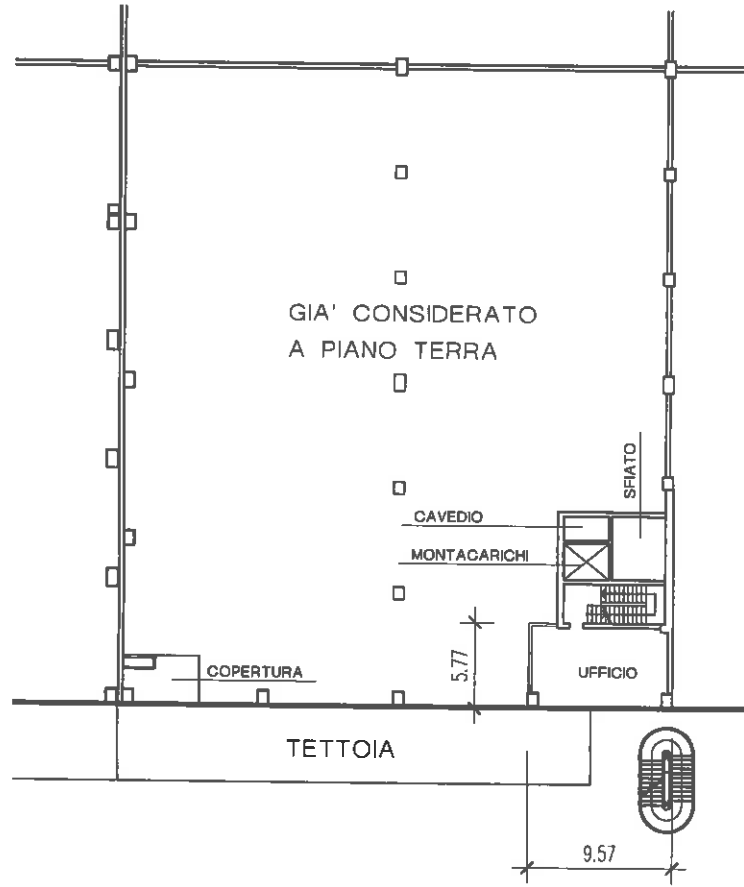
PRIMO PIANO H.m.= ml. 2.60
