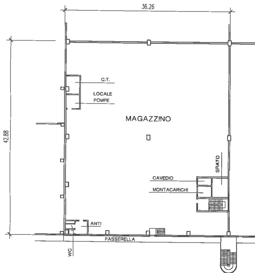
SECONDO PIANO H.m.= ml. 5.80
