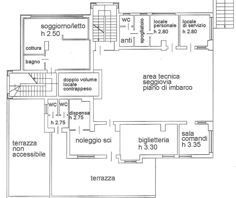
PIANO PRIMO
